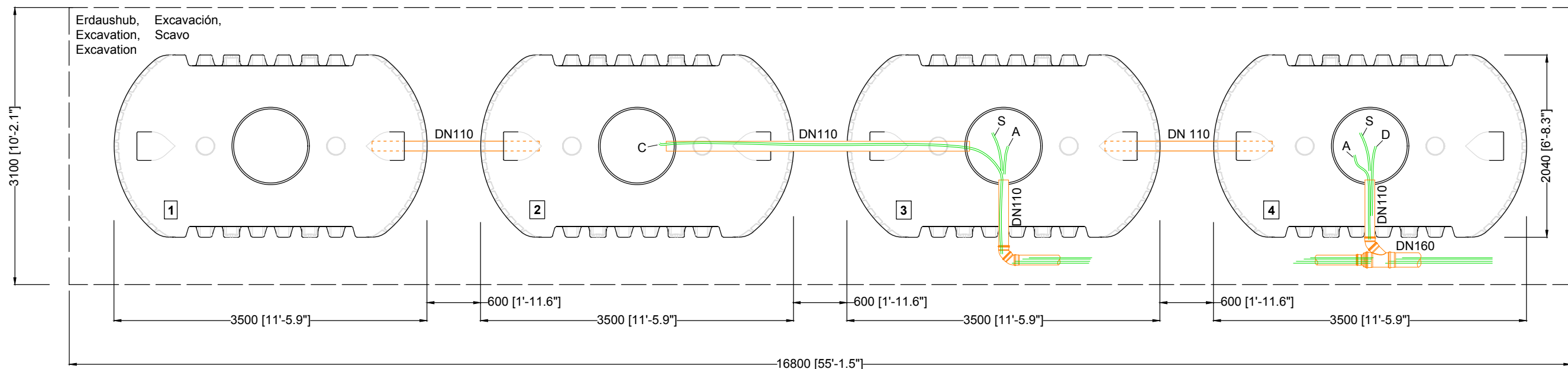
Grundriss Luftschläuche Top view compressed air Plan de raccordement des tuyaux d'air Vista superior tubería aire comprimido Pianta dei tubi di aria compressa
