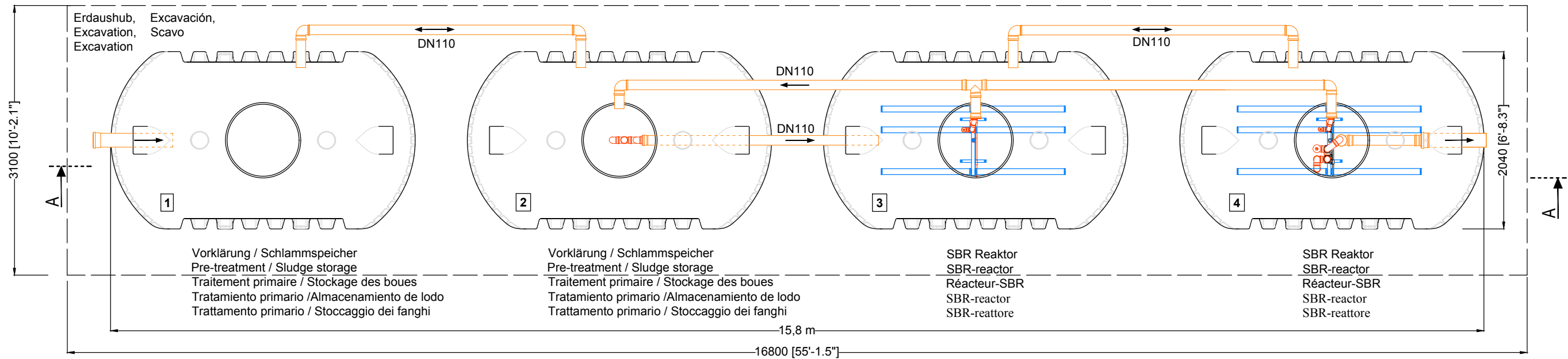
Grundriss Abwasserbehandlung Top view wastewater treatment Plan de mise en oeuvre Planta tratamiento de aguas residuales Pianta del trattamento delle acque reflue
